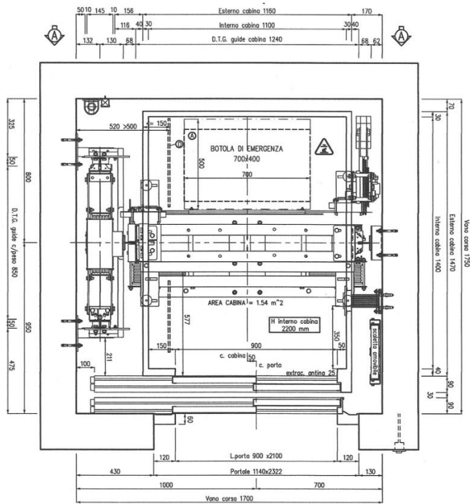
Dimensioni vano e cabina con meccanica a SX
